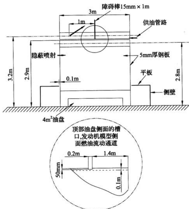
图 A. 3. 2-2 设备模型和试验设施布置
