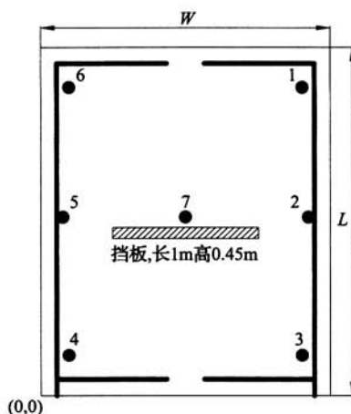
图 A.5.2-1 油罐火位置
