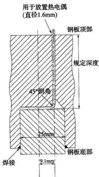
图 A. 2. 11-2 喷雾冷却试验热电偶布置
