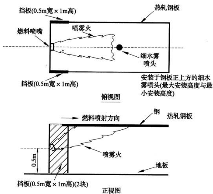
图 A. 2. 11-1 喷雾冷却试验布置
