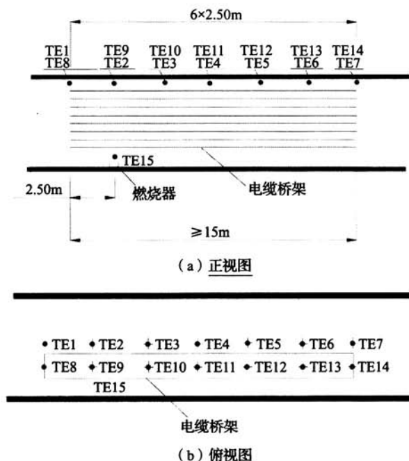
图 A.4.4 试验热电偶布置
