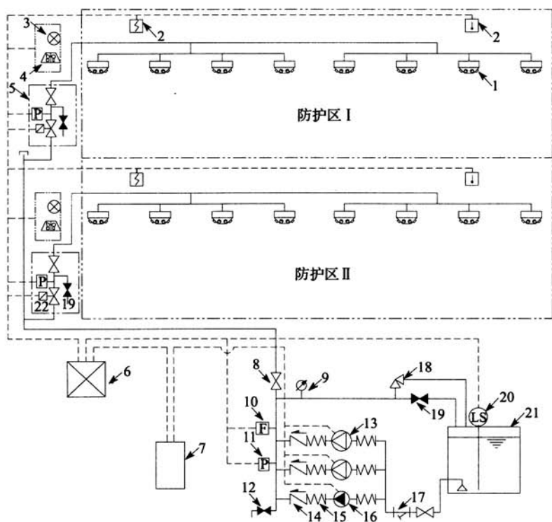
图 1 开式系统示意
