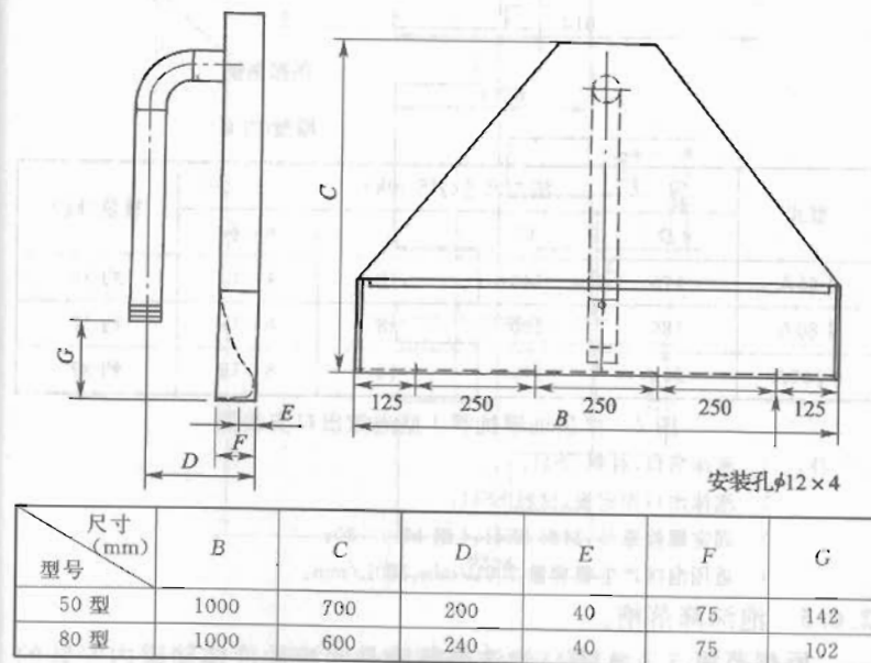
图 1 泡沫倾注器
