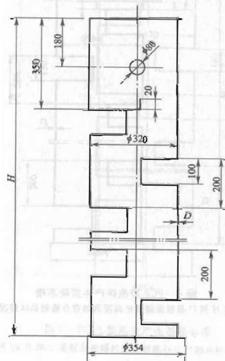
图3 PC4 型泡沫产生器降落槽
