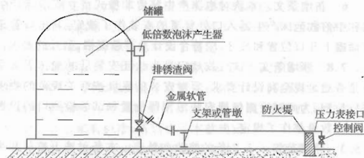
图 7 支架或管墩安装示意图
