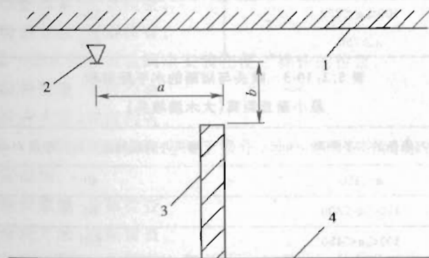
图 5.2.10 喷头与隔断障碍物的距离
